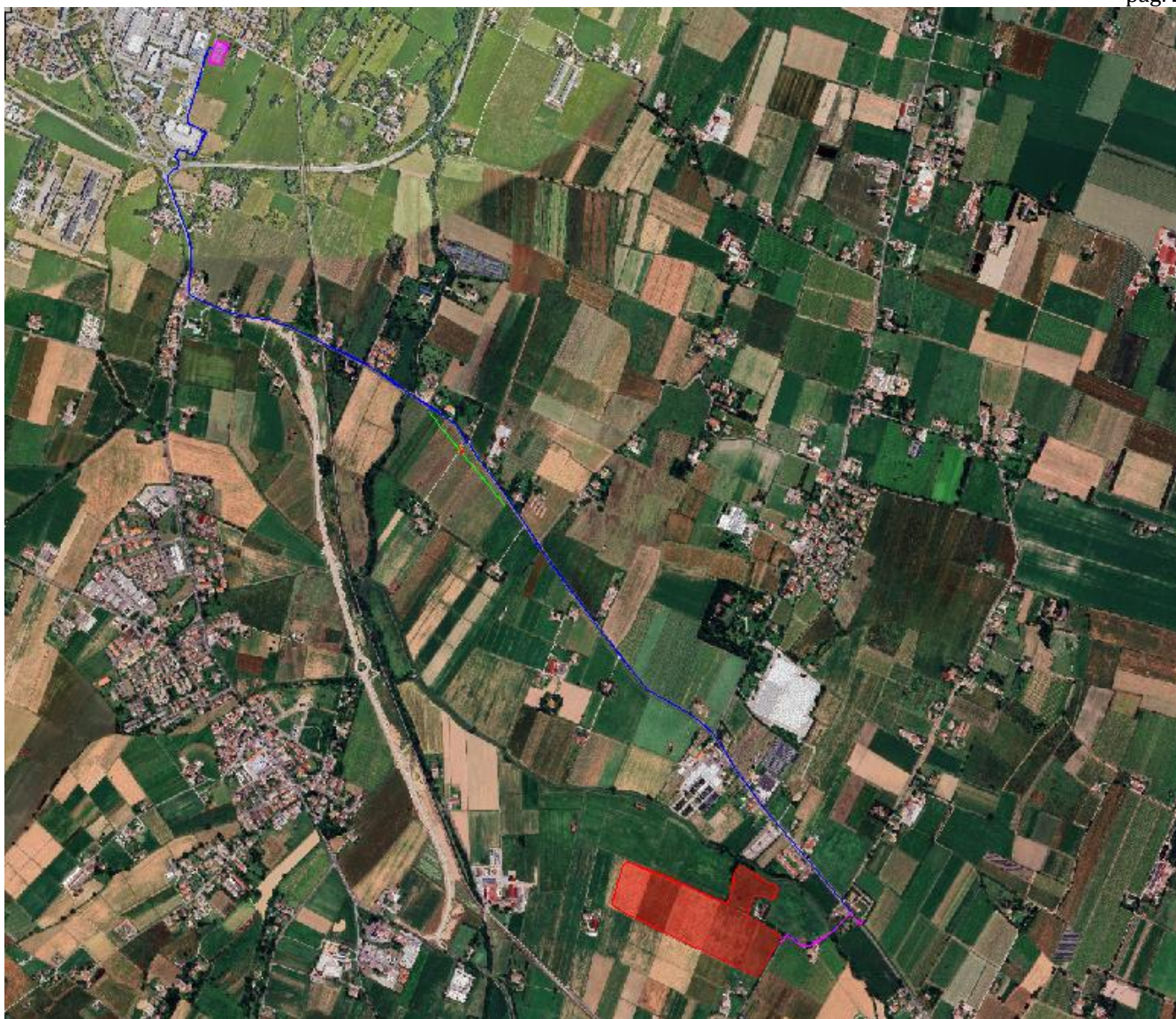
Figura 1 - Layout d'impianto e interconnessione
