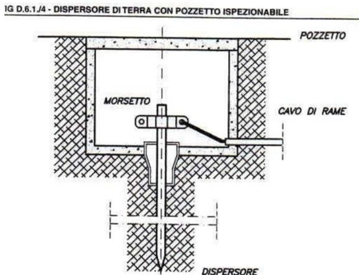
Figura 3-1 dispersore di terra con pozzetto ispezionabile
