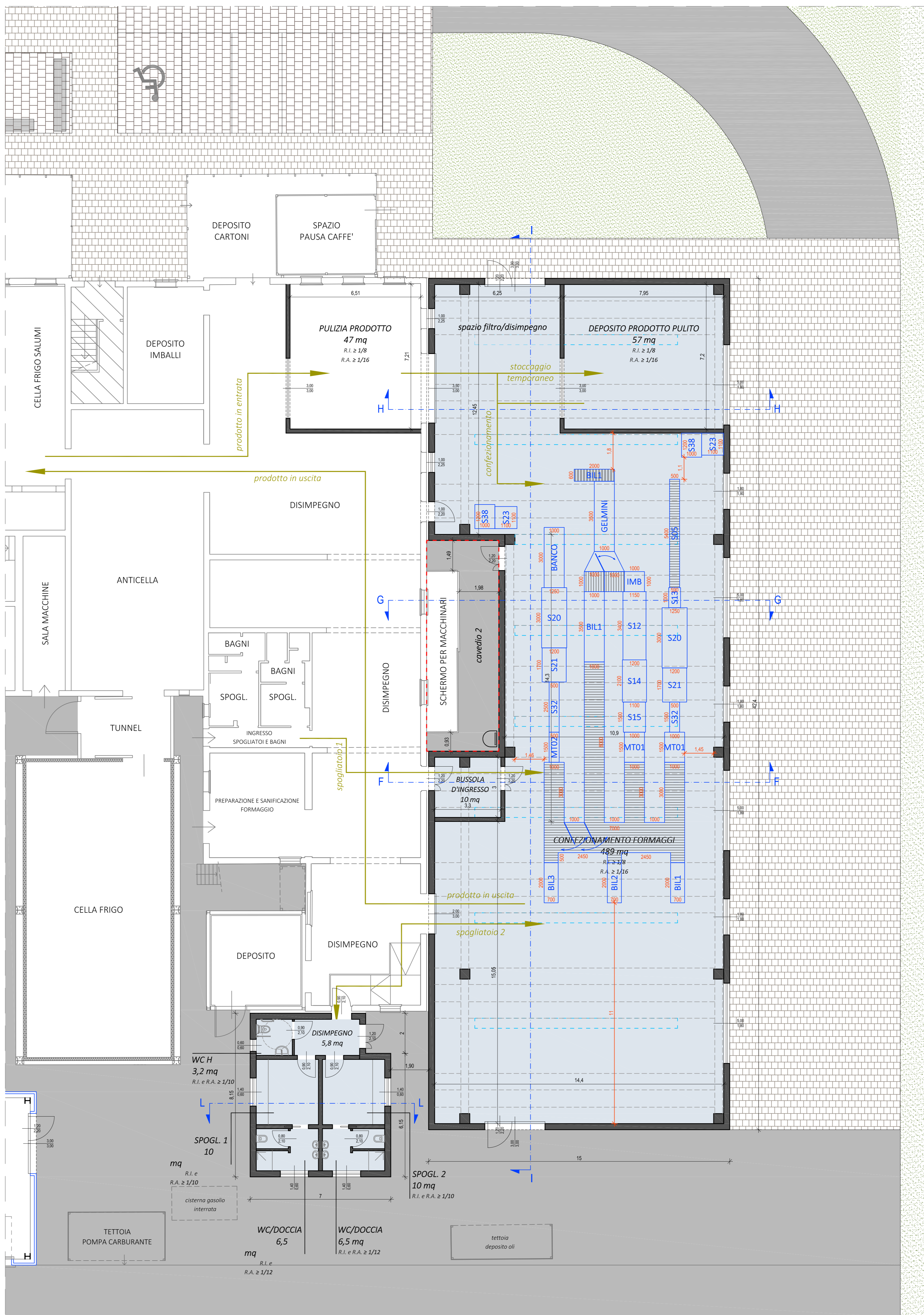
PIANTA PIANO TERRA Scala 1:100
