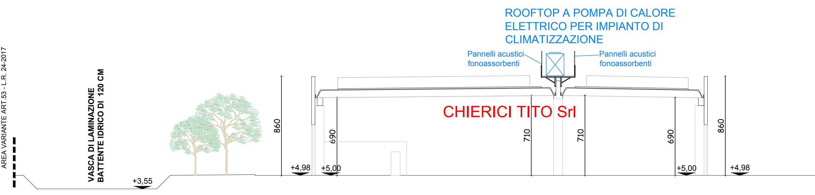
SEZIONE C-C
