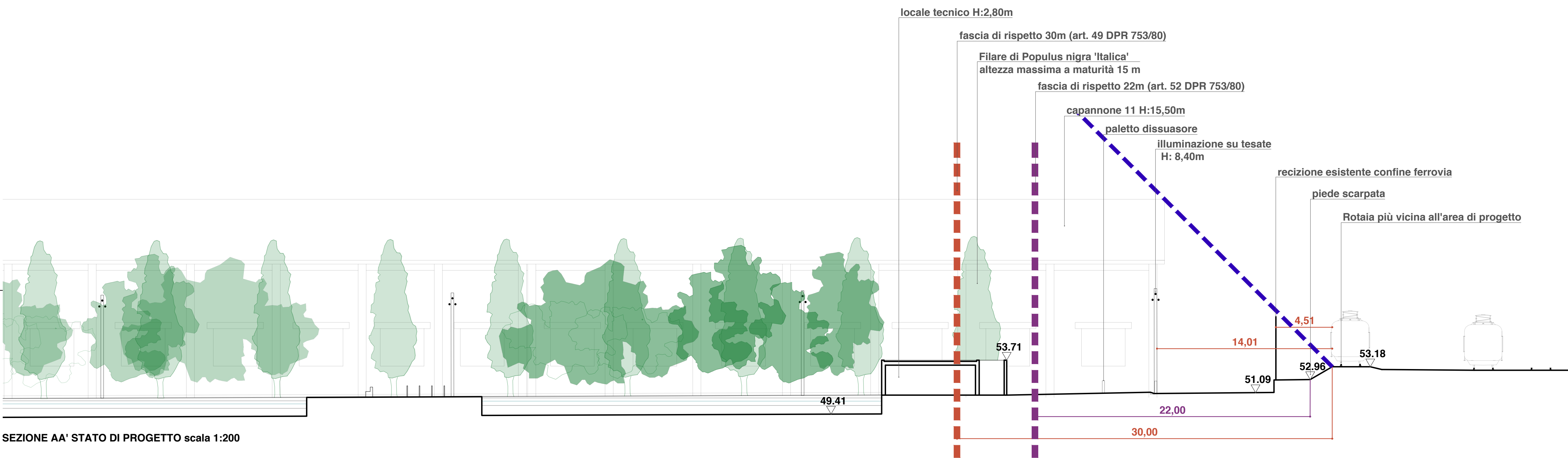
SEZIONE AA' STATO DI PROGETTO scala 1:200
