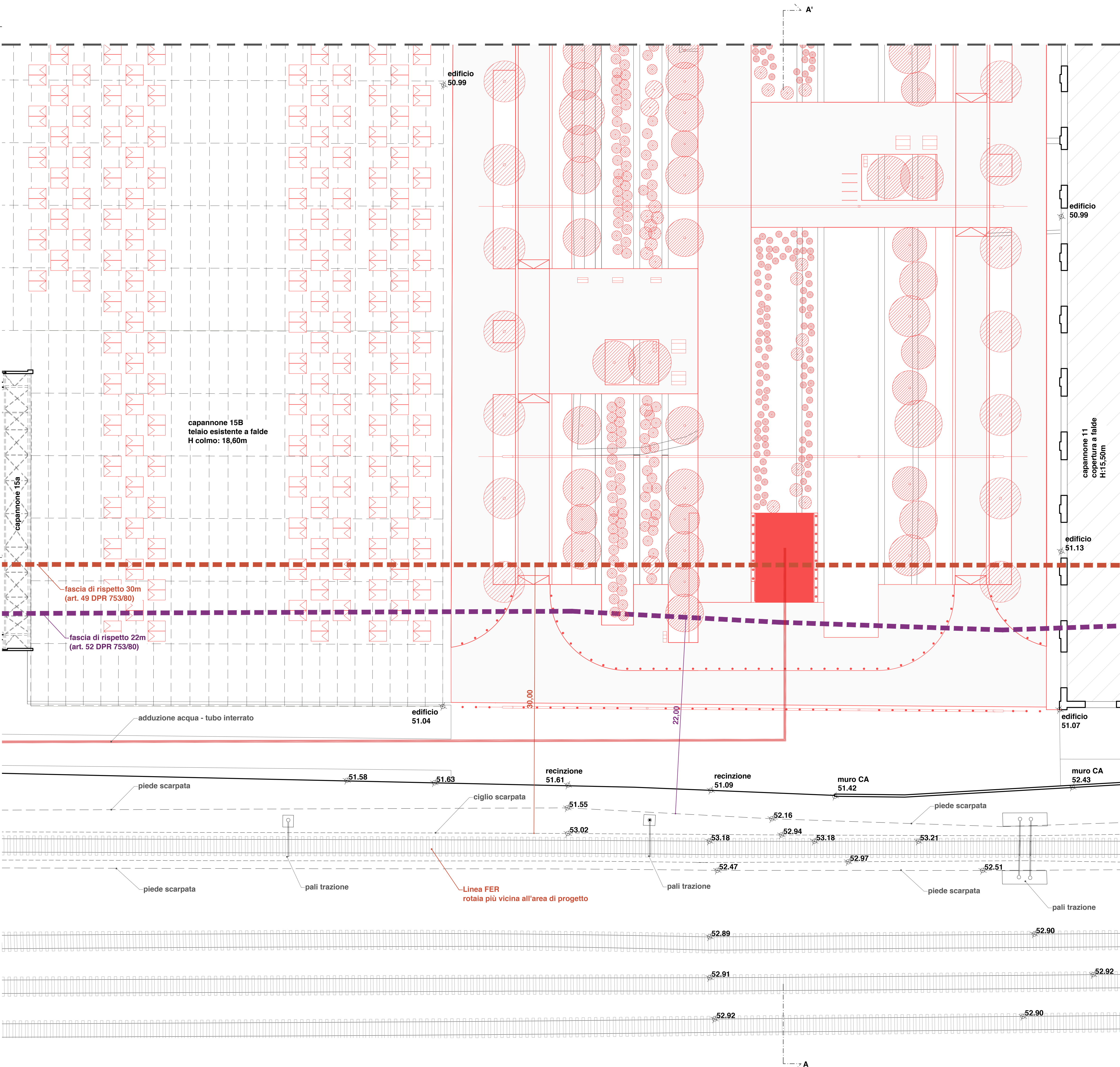
DETTAGLIO PLANIMETRIA SOVRAPPOSTO DEMOLIZIONI E COSTRUZIONI scala 1:200
