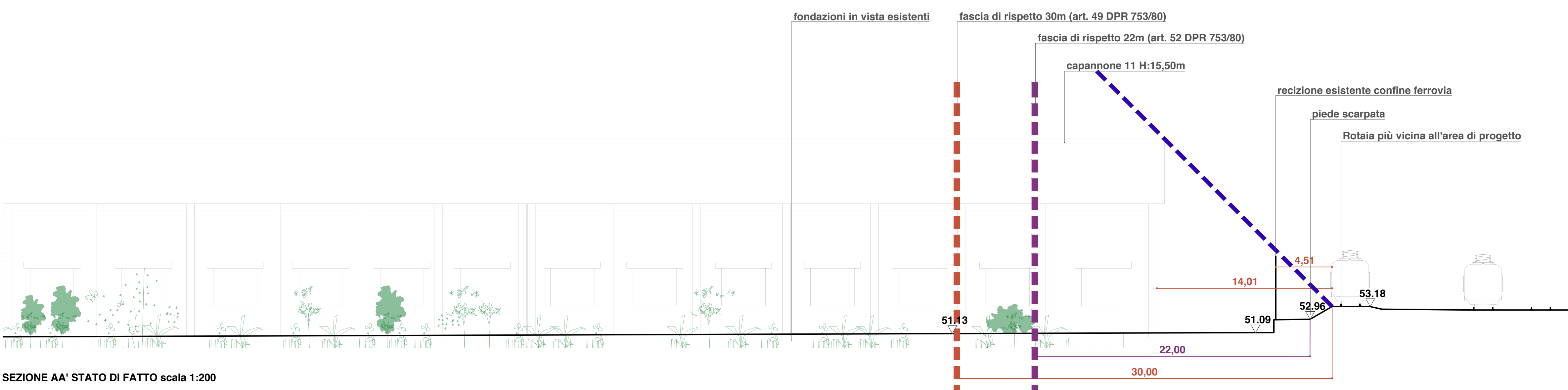
SEZIONE AA' STATO DI FATTO scala 1:200
