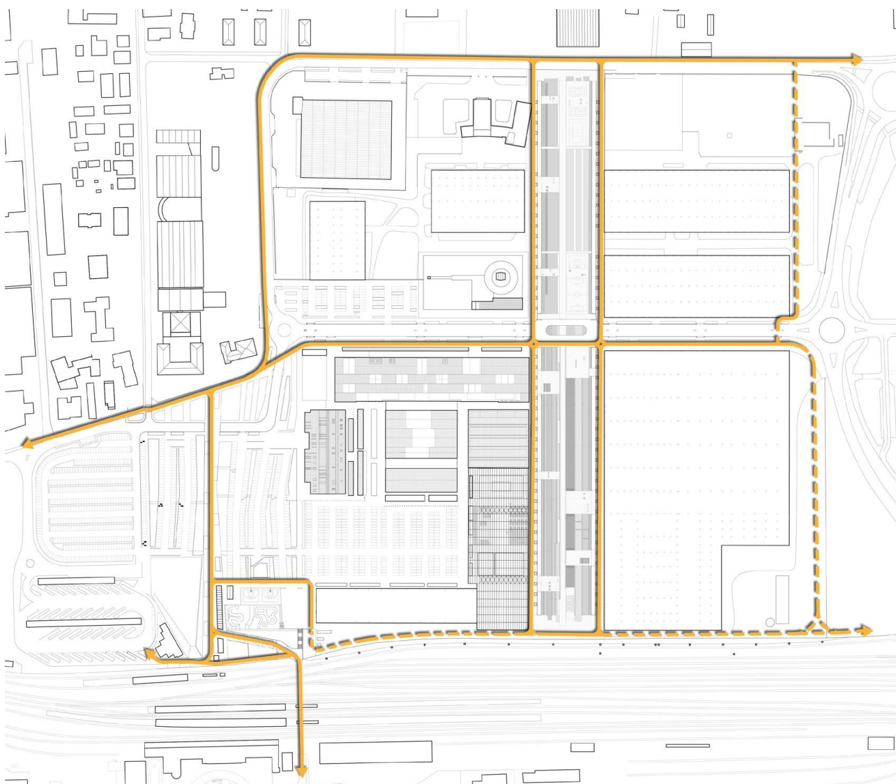
Figura 16 – Sistema della circolazione ciclopedonale.
