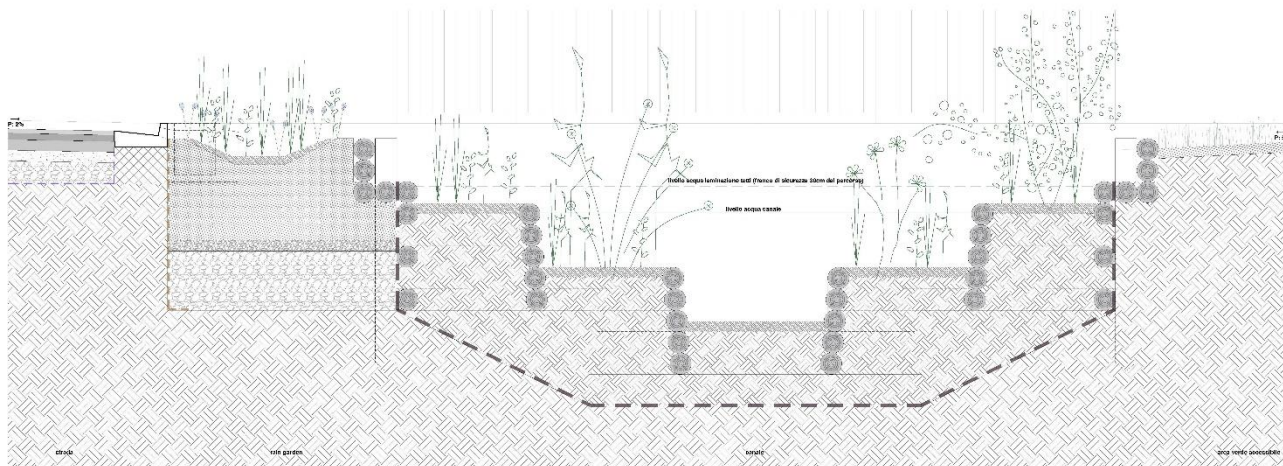
Figura 17 – Sezione del canale.
