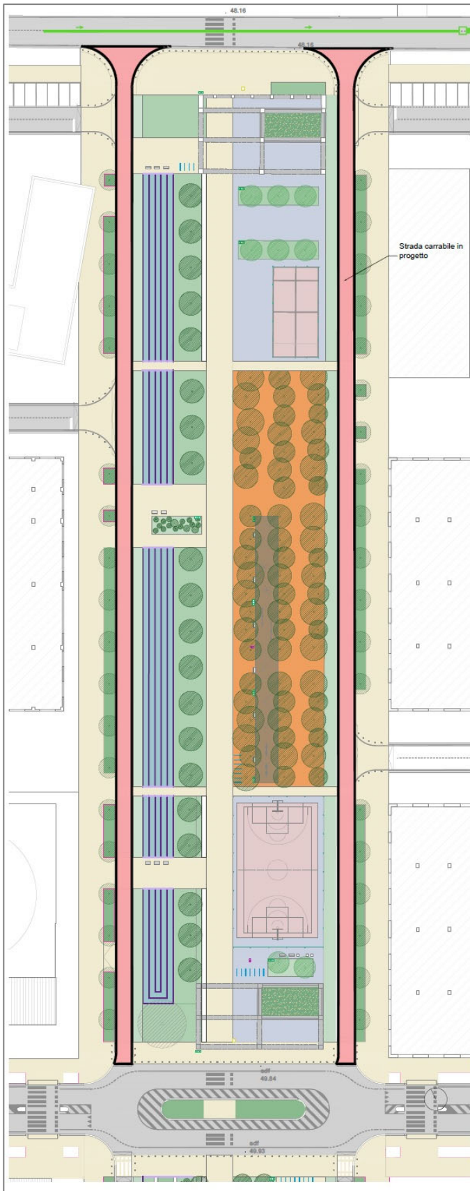
Figura 9 – Individuazione delle opere stradali (evidenziate in rosso) all'interno della Rambla Sud
