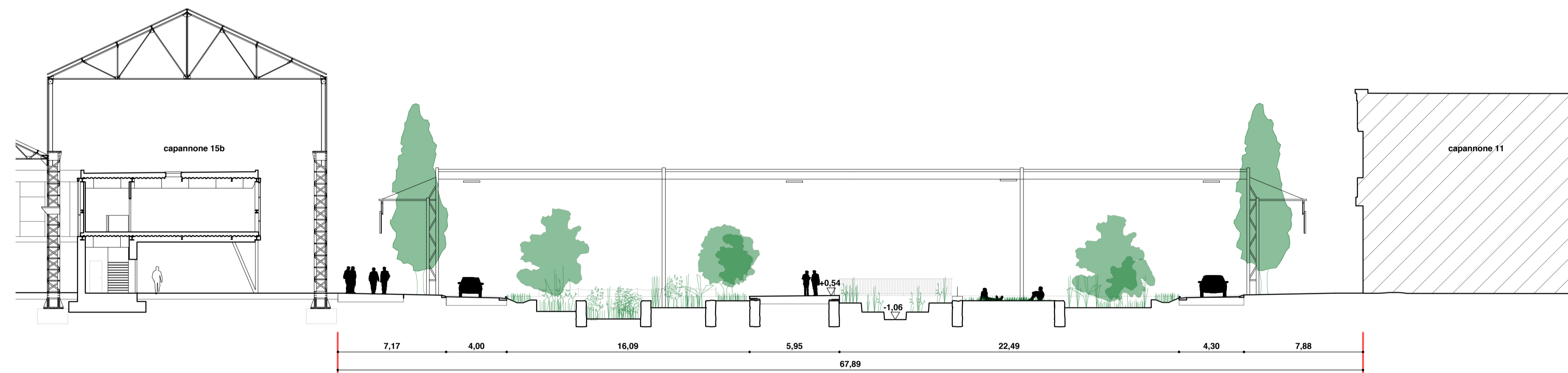
SEZIONE AA'
