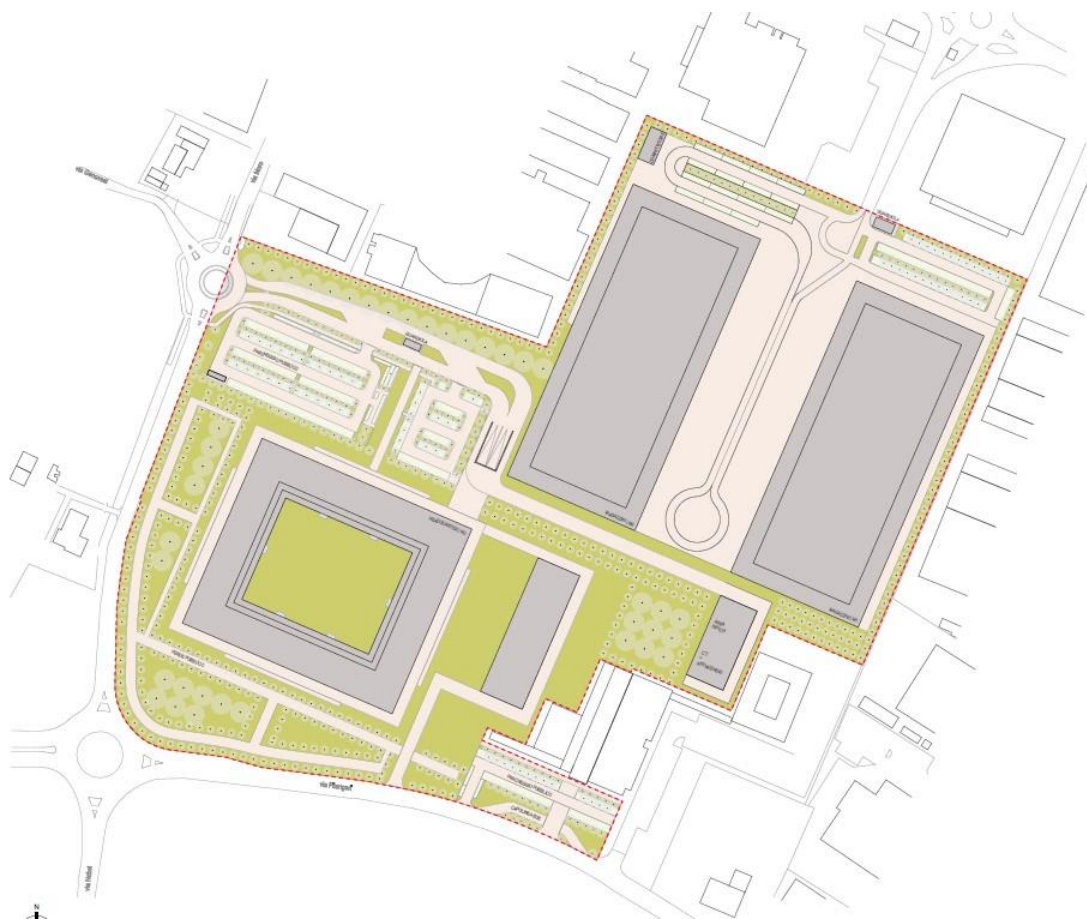
Progetto del nuovo comparto industriale
