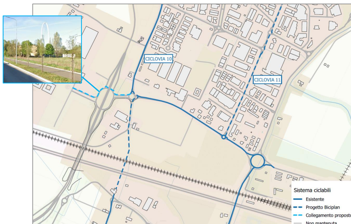
Ipotesi di collegamento ciclabile con l'headquarter esistente
