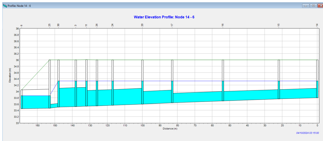
Profilo max riempimento dorsale principale
