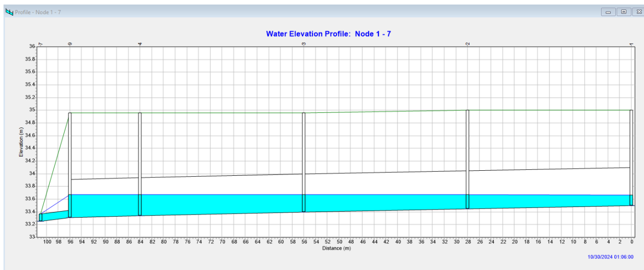
Profilo max riempimento collettore scat. 120x60 cm
