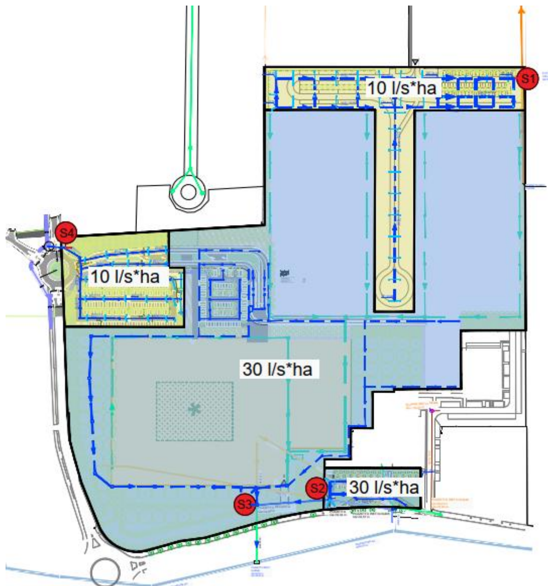
Planimetria con inquadramento dei bacini di progetto e dei quattro punti di recapito S1÷S4
