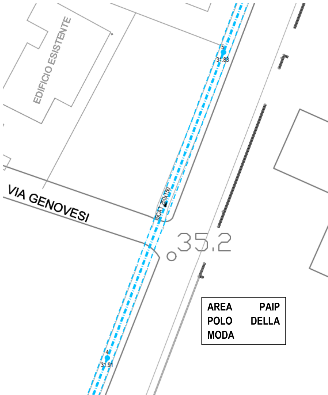
Planimetria progetto - tombamento Cavo Baggiovara Via Moro zona recapito nuovo parcheggio
