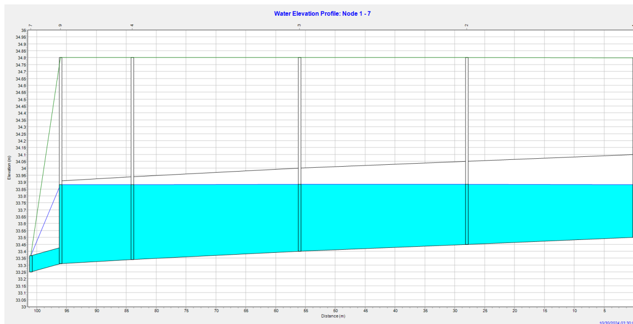
Profilo collettore principale strada – Massimo livello in corrispondenza del picco di pioggia
