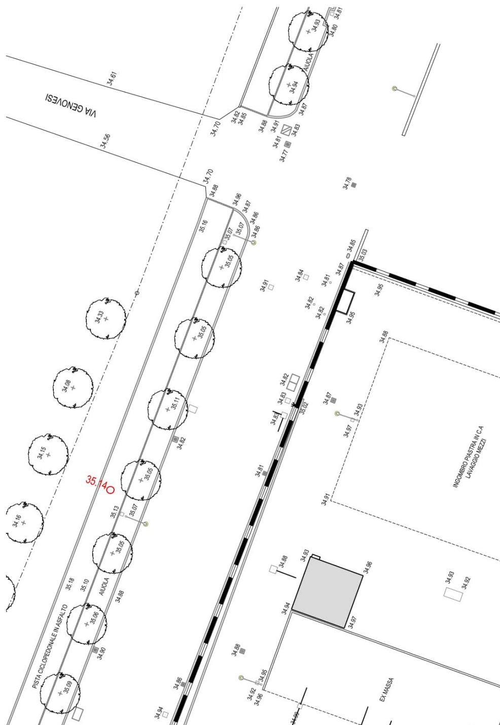
Rilievo topografico - tombamento Cavo Baggiovara Via Moro zona recapito nuovo parcheggio
