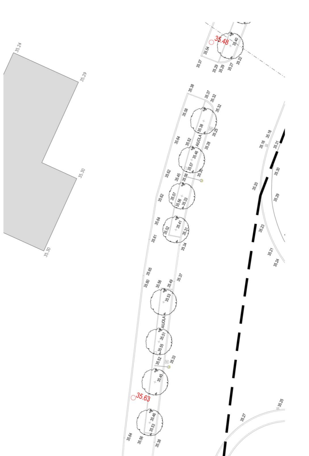
Rilievo topografico - inizio tombamento Cavo Baggiovarena
