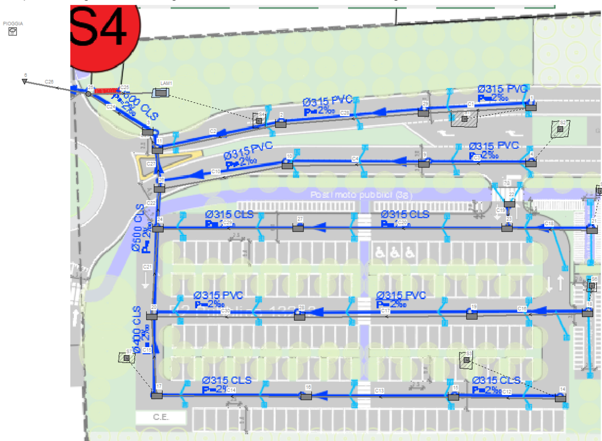
Modello di calcolo opere di urbanizzazione Via A. Moro
