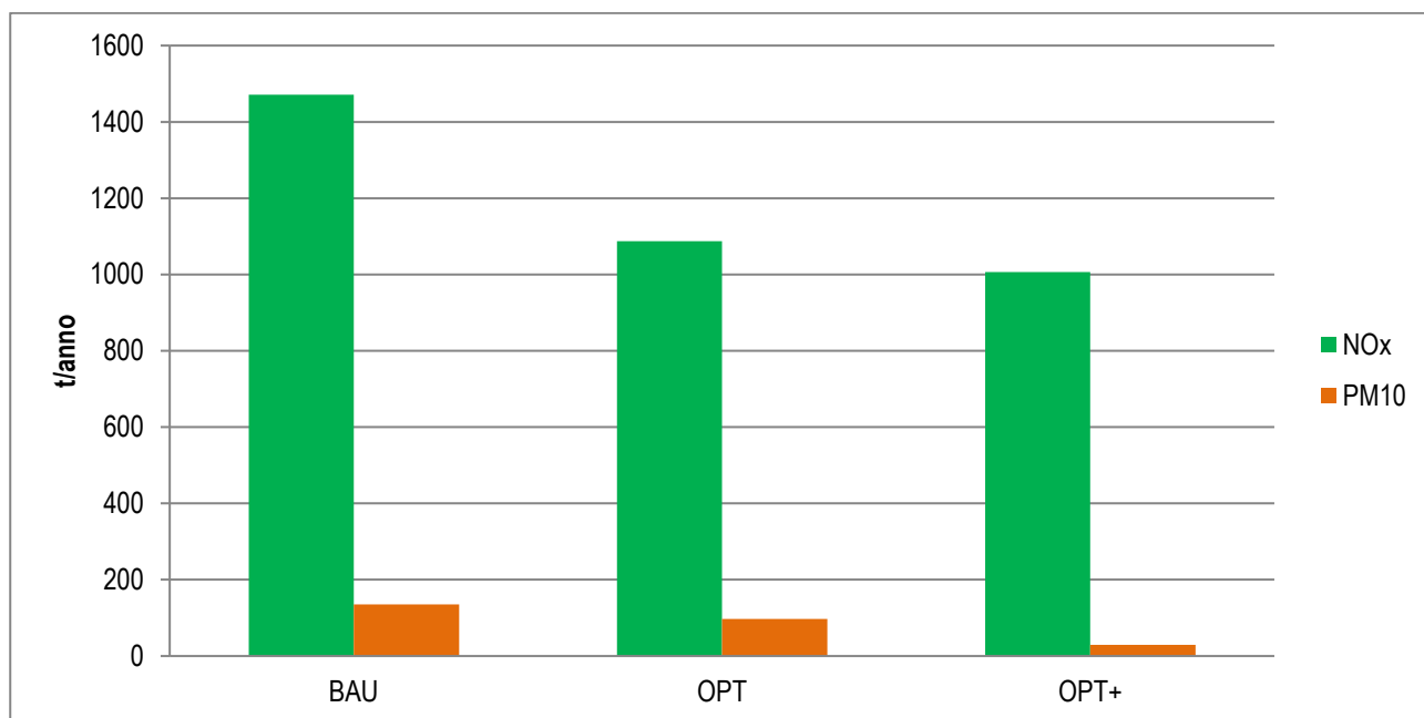
Figura 12: Grafico di confronto dei tre scenari emissivi
