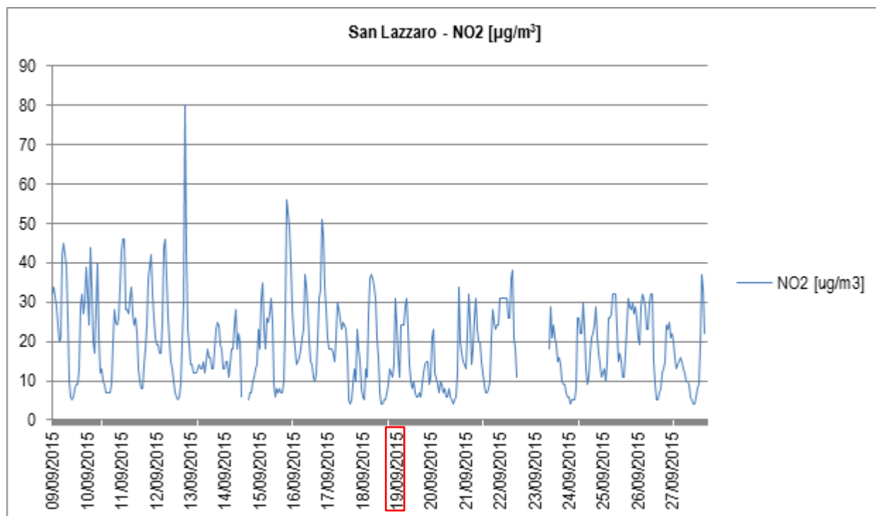
Figura 21: Concentrazioni emissive medie orarie di NO 2 – Stazione San Lazzaro (Settembre 2015)
