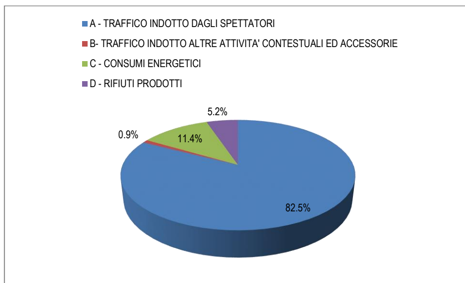
Figura 26: Grafico di distribuzione percentuale dei contributi di CO 2eq per le attività connesse all'esercizio dell'Arena Eventi
