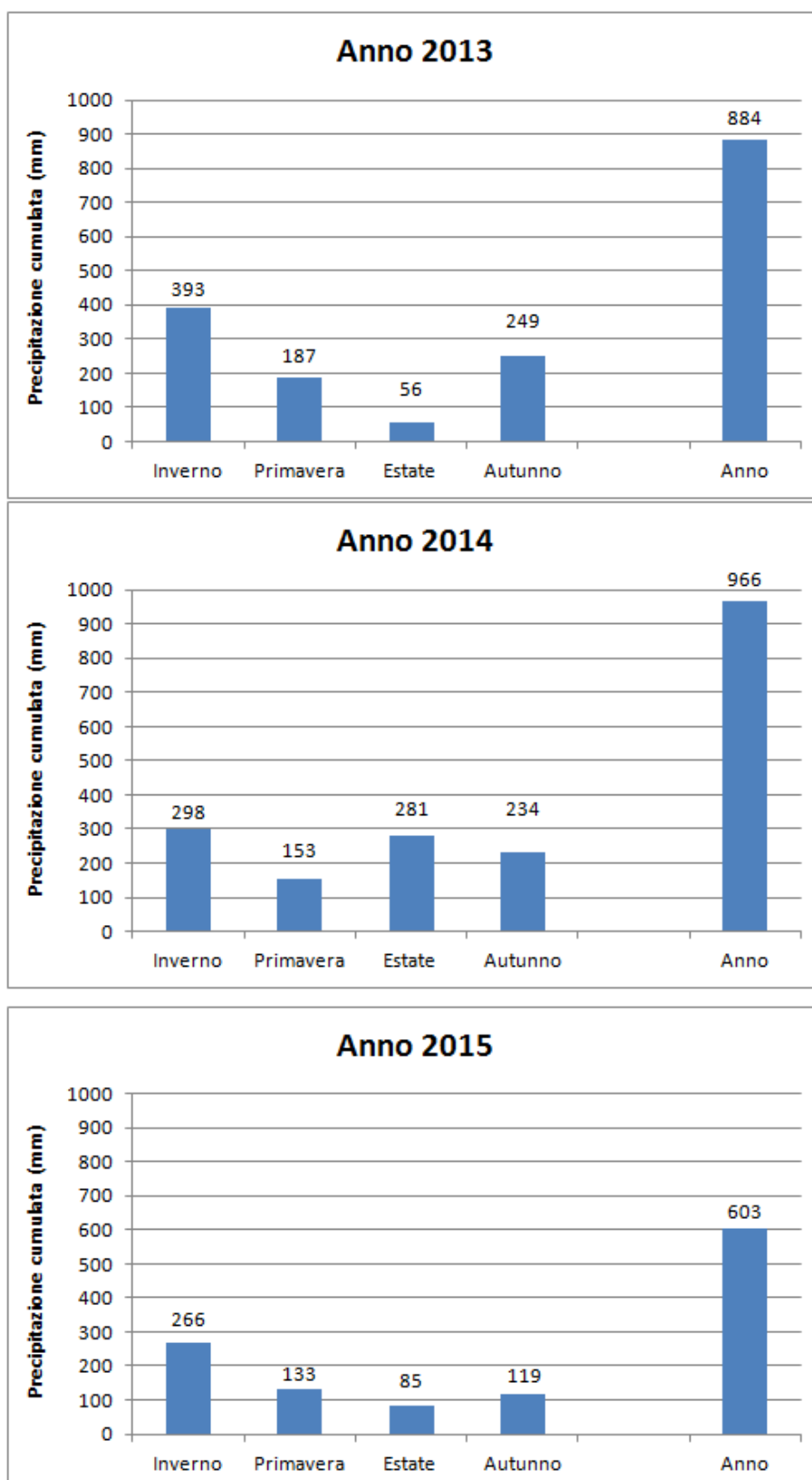
Figura 2: Precipitazioni registrate dalla stazione di Reggio Emilia negli anni 2013, 2014 e 2015
