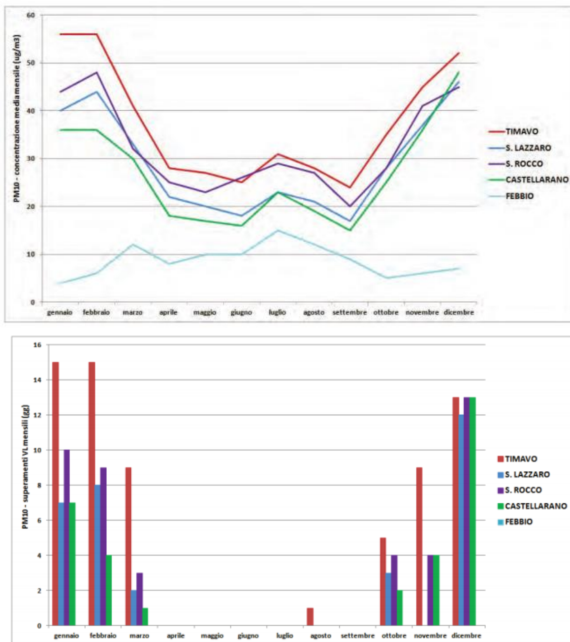
Figura 14: Concentrazioni medie mensili e giorni di superamento per il PM10 nel 2015 (ARPAE RE)
