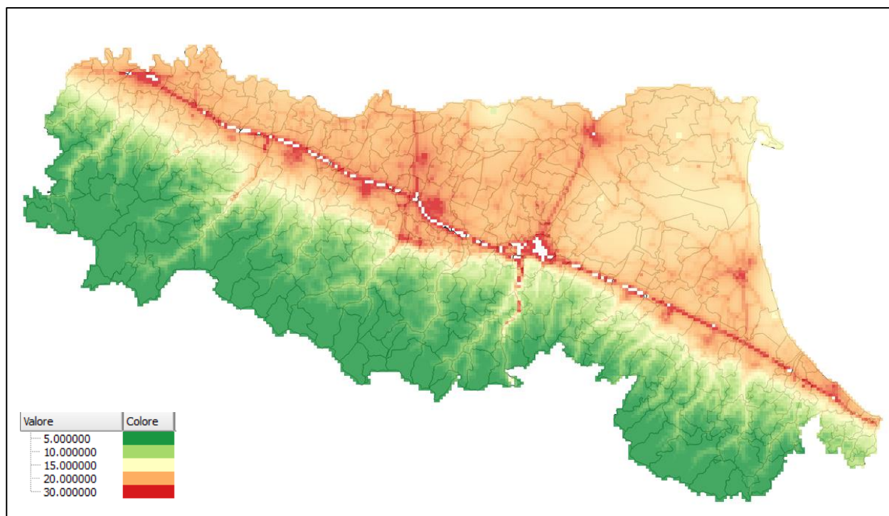
Figura 8: Concentrazioni di Fondo NO 2 (valore medio annuo 2015 \mu\text{g}/\text{m}^3 ) – Fonte dataset ARPAE, nostra rielaborazione
