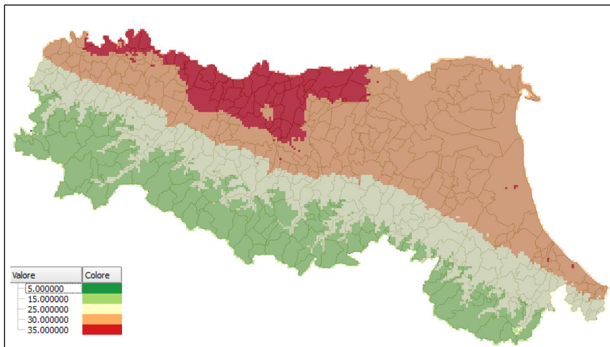
Figura 9: Concentrazioni di Fondo PM 10 (valore medio annuo 2015 \mu\text{g}/\text{m}^3 ) – Fonte dataset ARPAE, nostra rielaborazione
