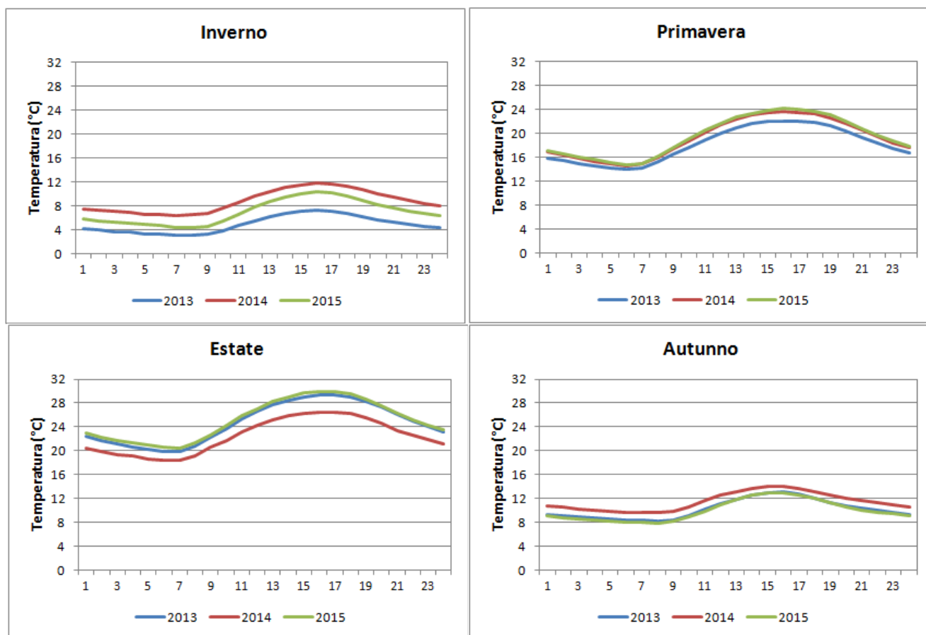
Figura 1: Grafici dell'andamento del giorno tipo dei valori di temperatura (stazione di Reggio Emilia).
