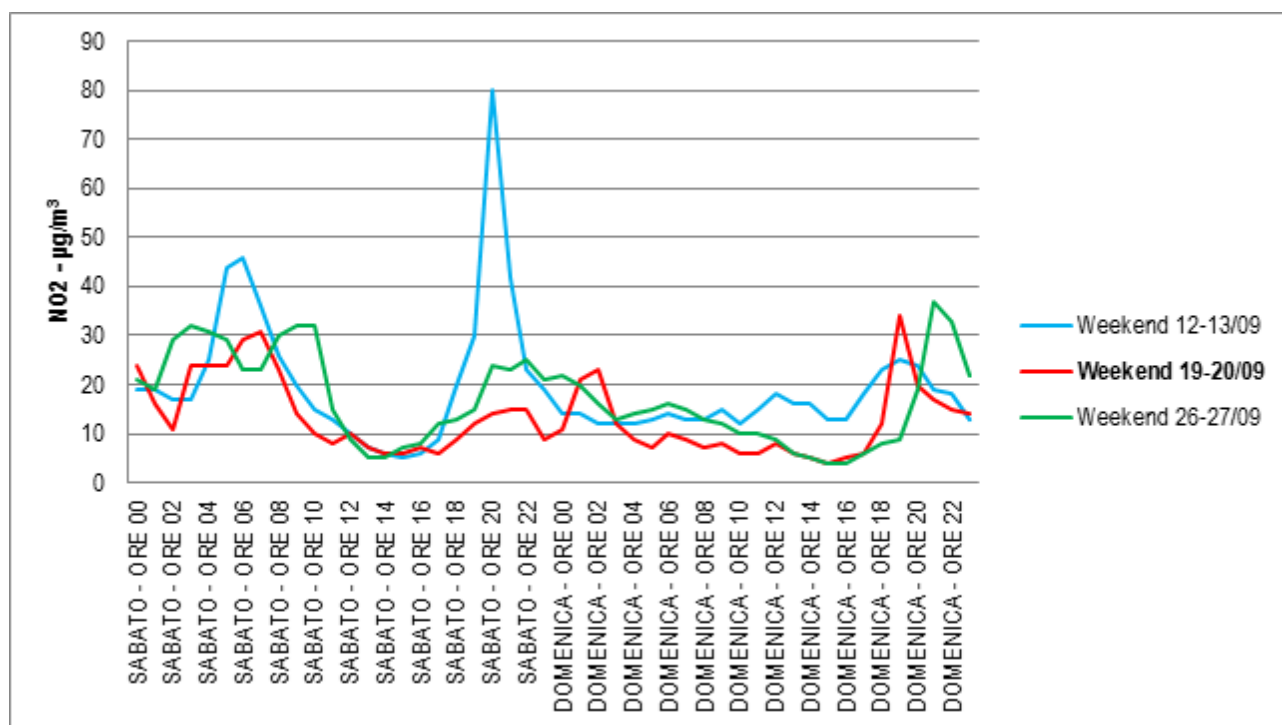
Figura 22: Confronto concentrazioni medie orarie di NO 2 per tre weekend W1, W2 e W3 in merito al concerto Campovolo 2015 (W2 – linea rossa)
