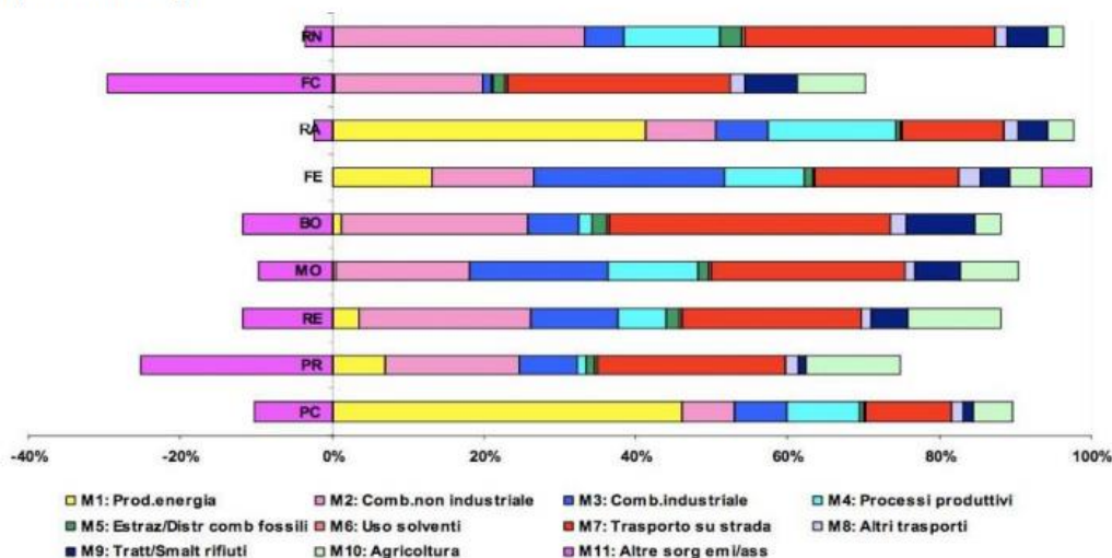
Figura 25: Distribuzione percentuali delle emissioni e degli assorbimenti di CO2 in Emilia Romagna, per macrosettore (kt/anno)
