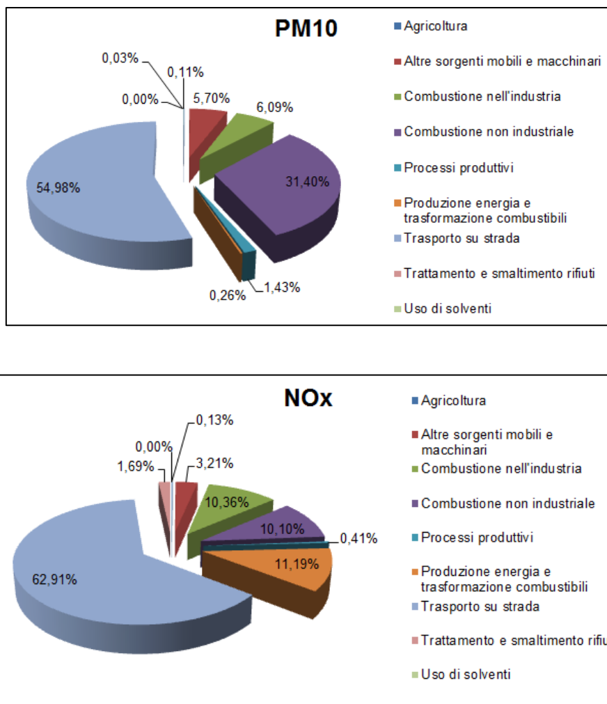
Figura 13: Grafici emissioni PM10 ed NOx suddivise per macrosettore – Comune di Reggio Emilia – INEMAR 2010
