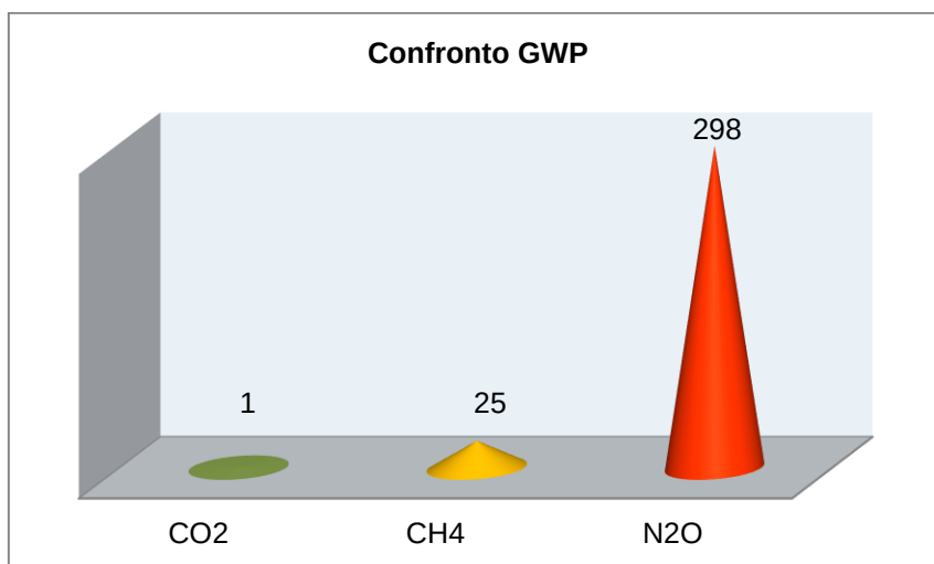
Figura 24: confronto tra global warming potential di CO2, CH4 e N2O
