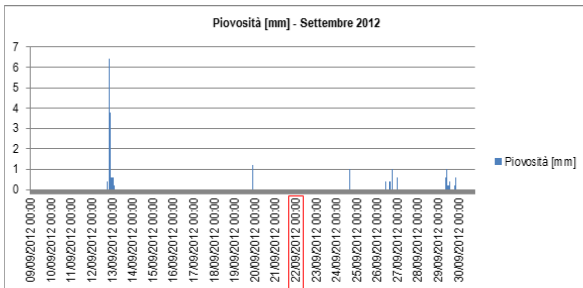
Figura 16: Condizioni meteorologiche di piovosità – settembre 2012
