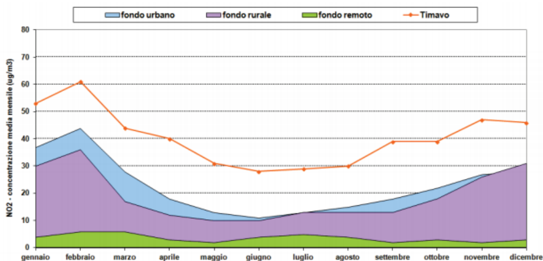
Figura 15: Concentrazioni medie mensili e giorni di superamento per il NO2 nel 2015 (ARPAE RE)
