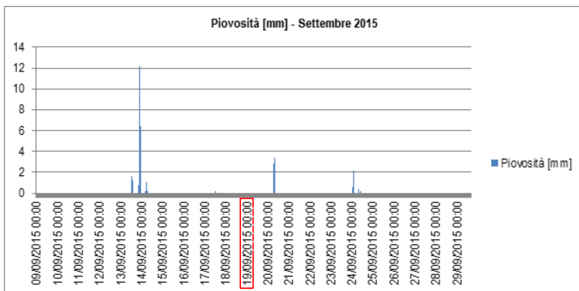
Figura 19: Condizioni meteorologiche di piovosità – settembre 2015
