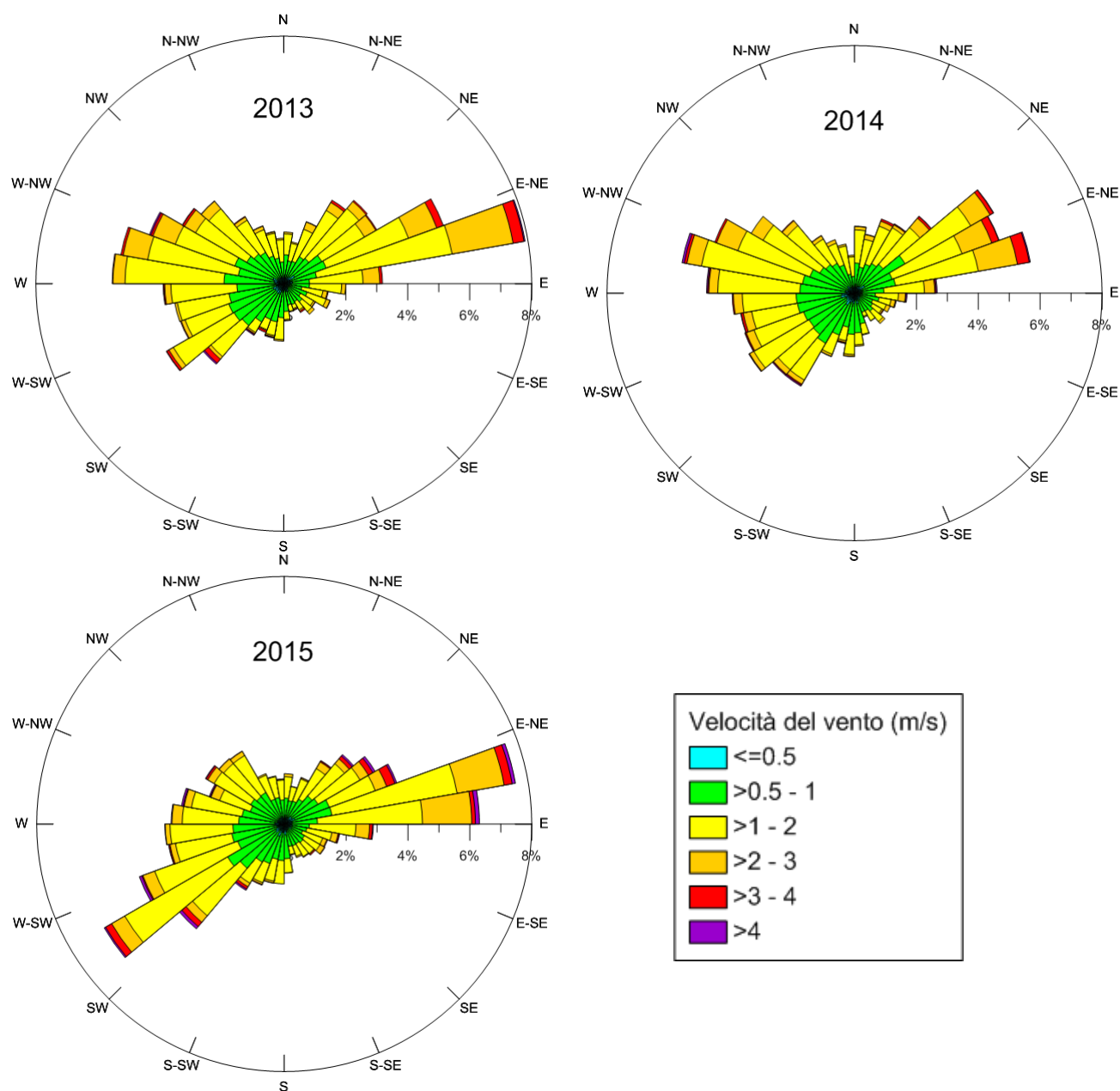
Figura 3: Rose dei venti a 10 m di quota elaborate per Reggio Emilia (Anni 2013, 2014 e 2015)
