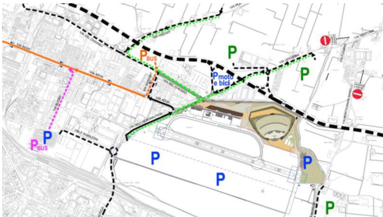
Figura 11: Stralcio planimetria area di parcheggio autobus
