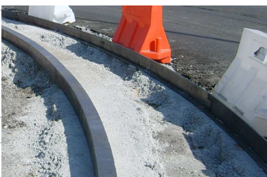
Cordolo in corten, nuova rotatoria di Mancasale (RE)
